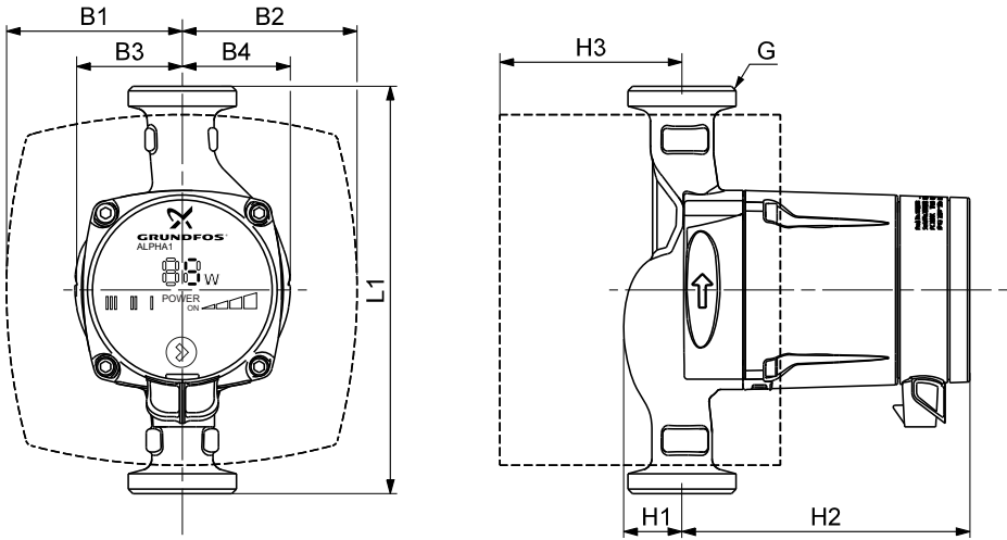
17. ábra Méretezett rajzok, ALPHA1 XX-40, XX-45, XX-60
