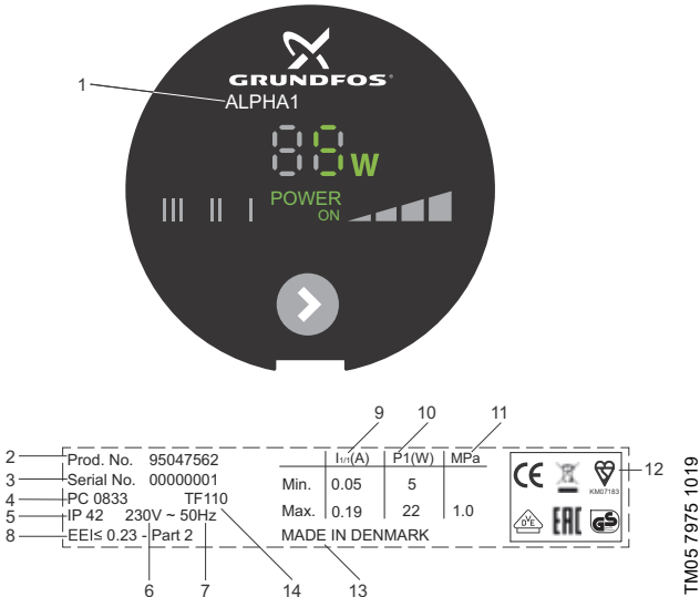
8. ábra Példa az adattáblára
