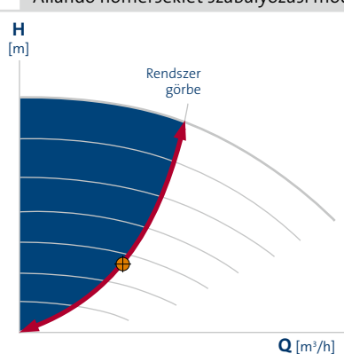
Állandó hőmérséklet szabályozási mód
