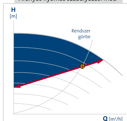
Arányos nyomás szabályozási mód
