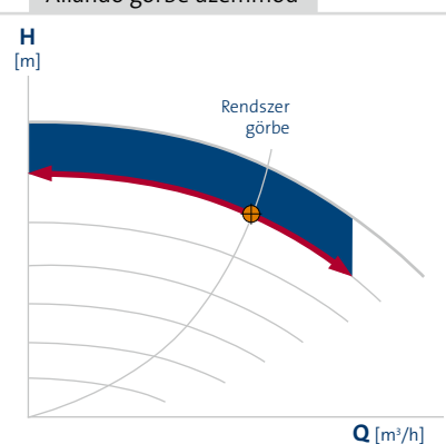
Állandó görbe üzem mód
