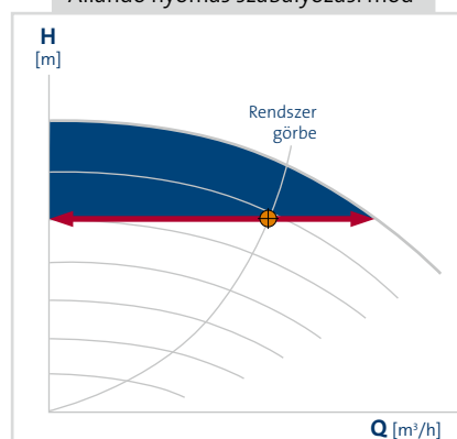
Állandó nyomás szabályozási mód
