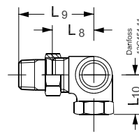
Térsarok szelep
