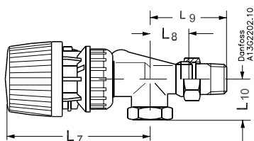
Fordított sarokszelep RA 2990 érzékelővel
