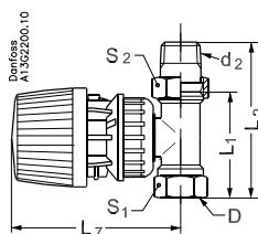
Egyenes szelep RA 2990 érzékelővel
