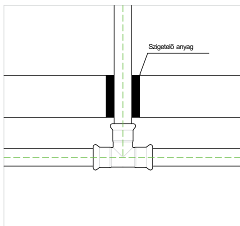
Födémáttörés alatti csővezeték
