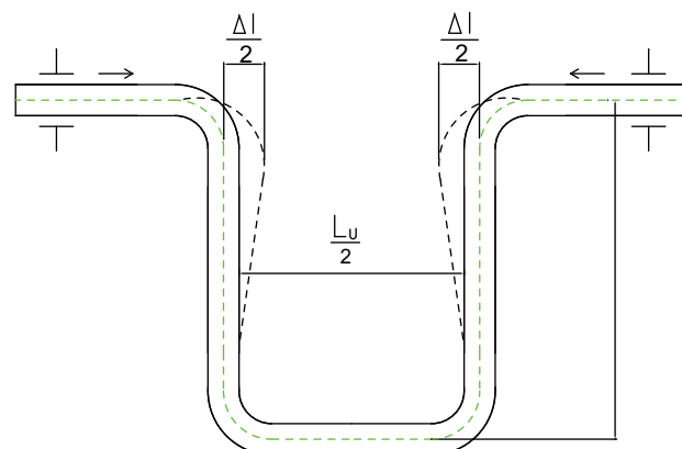
A vezetékből kialakított U-íves kompenzátor
