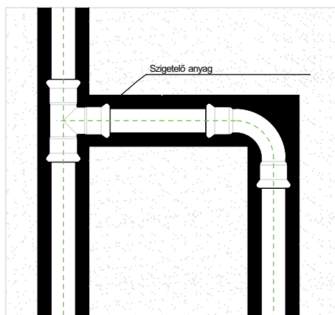
Falhoronyba fektetett csővezeték
