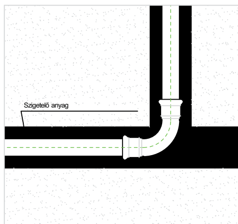
Úsztatott esztrich beton alá fektetett csővezeték
