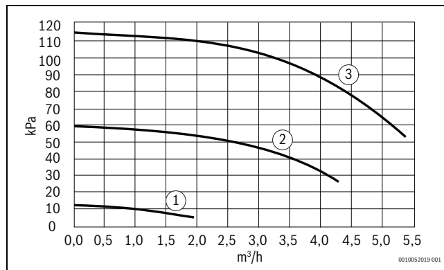
13. ábra CS2000AWF 18-30 R-T
