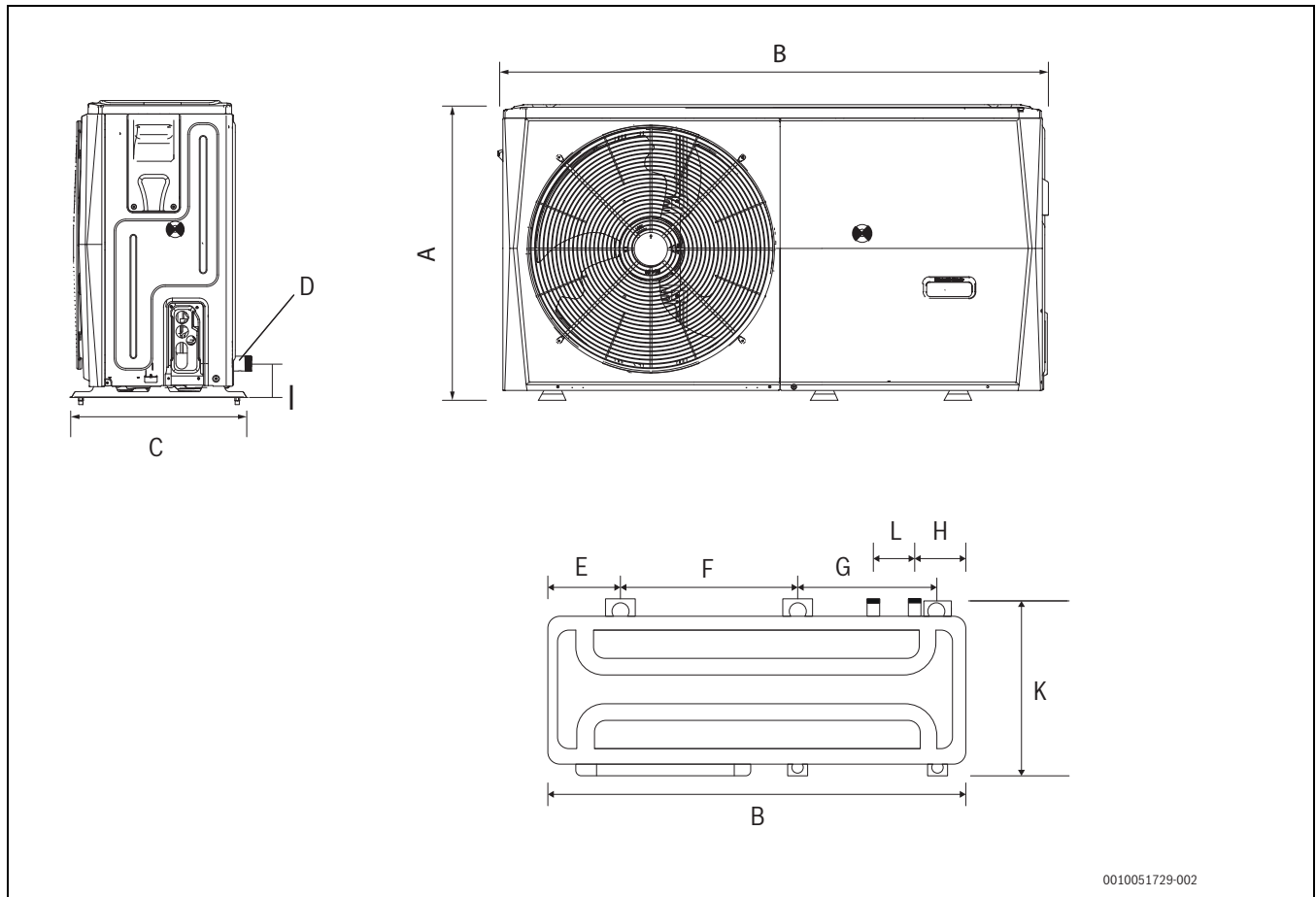
31. ábra CS2000AWF 4 R-S és CS2000AWF 6 R-S közötti méretek
