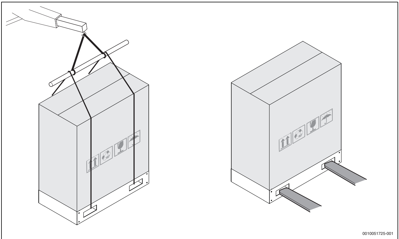
27. ábra Moztatás villástargonccal
