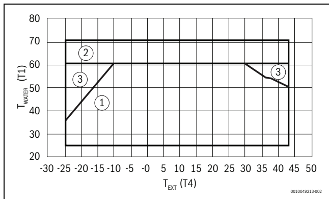
9. ábra CS2000AWF 18-30 R-T
