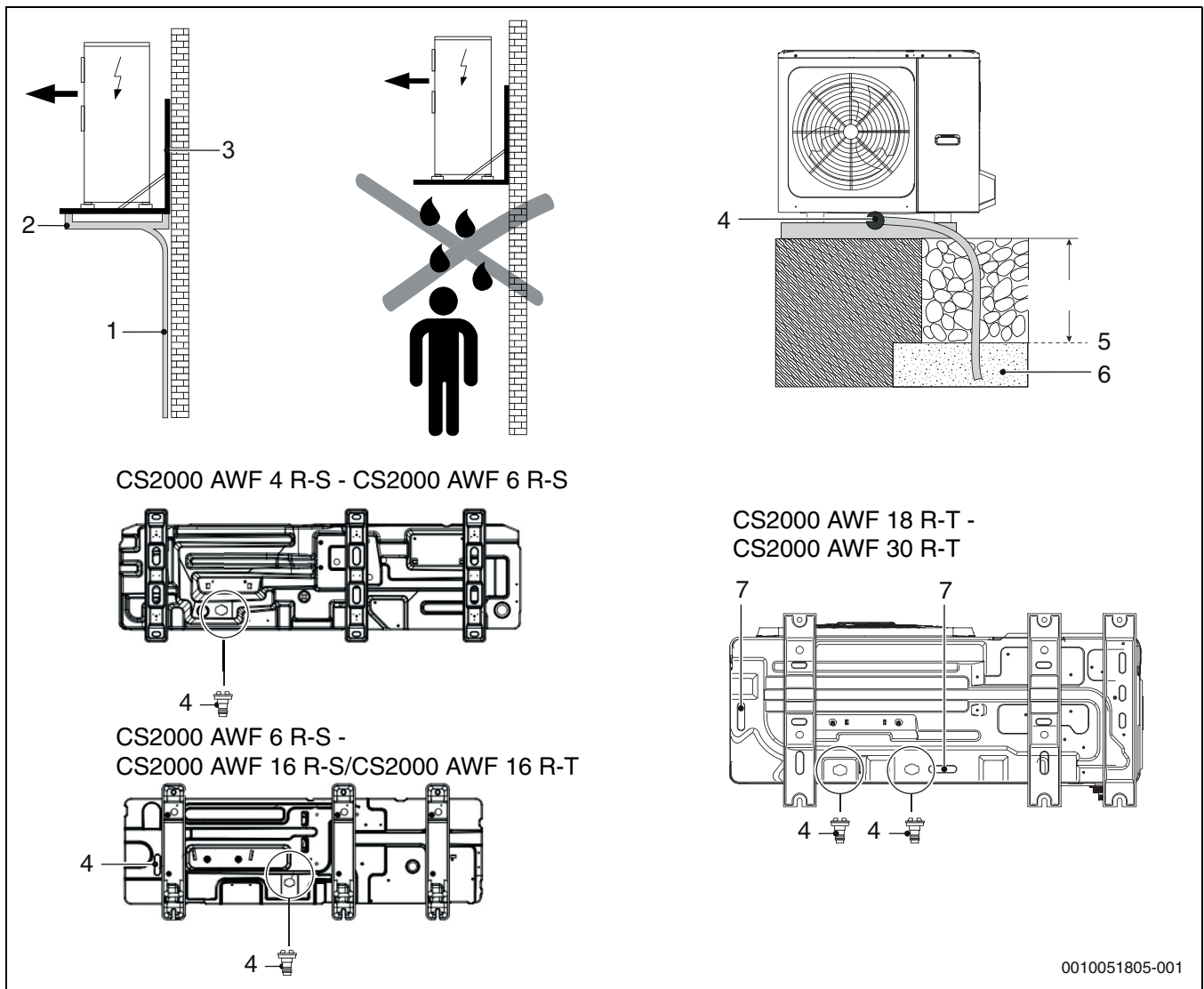
48. ábra Kondenzvíz-lefolyó
