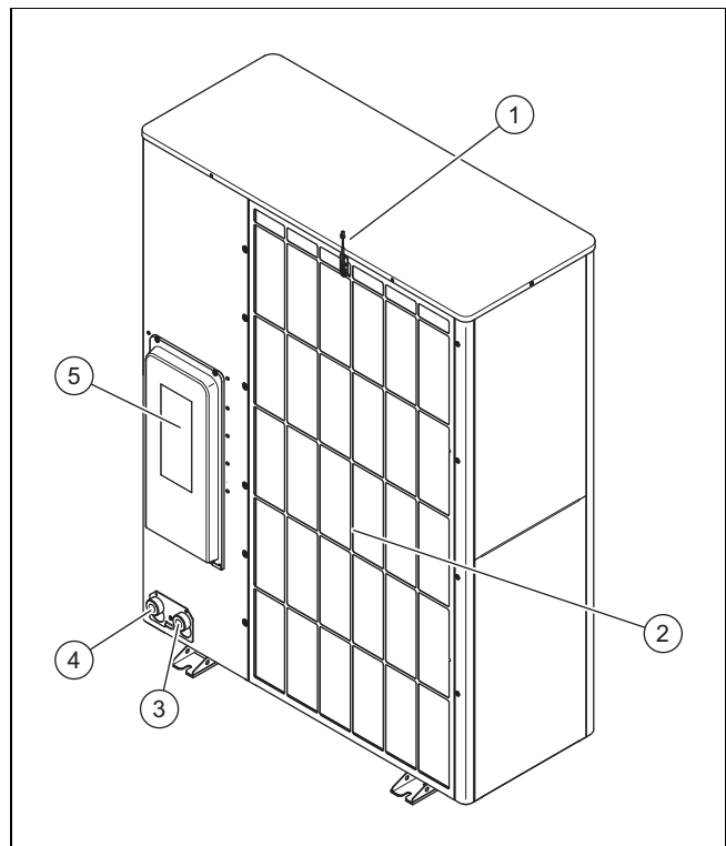
1 Датчик температури на вході повітря 4 Підключення до зворотної лінії системи опалення 2 Решітка входу повітря 5 Обшивка електричних підключень 3 Підключення до лінії подачі системи опалення
