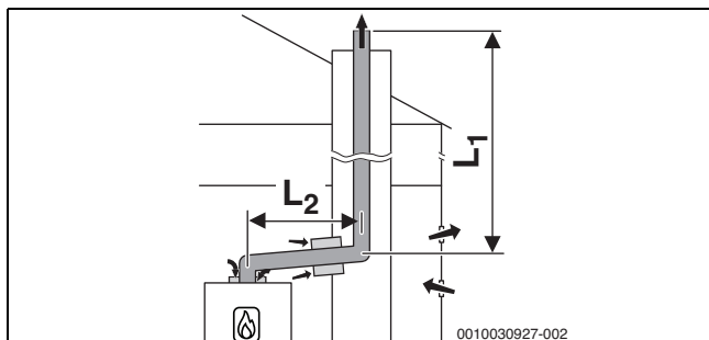
17. ábra B 23p /B 53p szerinti merev füstgázvezetés aknában, helyiség levegőtől függő levegőbevezetéssel a készülékbe és koncentrikus összekötő darabbal a felállítási helyiség és az akna között
