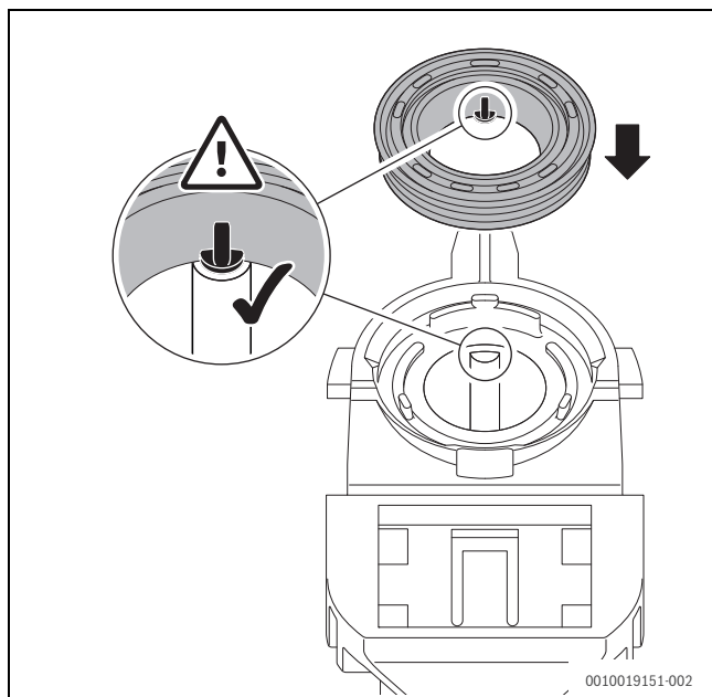
71. ábra Az új tömités beállítása a kondenzvízszfifonon
