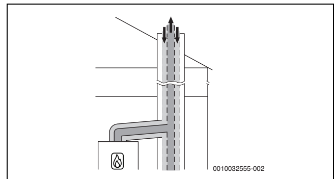
11. ábra A C 43x szerinti koncentrikus levegő-/füstgázvezetés a felállítási helyiségben
