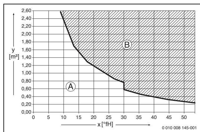
22. ábra A töltő- és pótvízzel szemben támasztott követelmények °fH-ban 50 kW teljesítmény alatti készülékeknél
