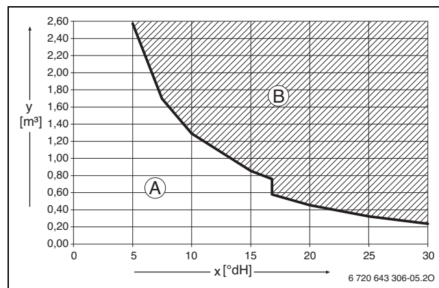
21. ábra A töltő- és pótvízzel szemben támasztott követelmények °dH-ban 50 kW teljesítmény alatti készülékeknél
