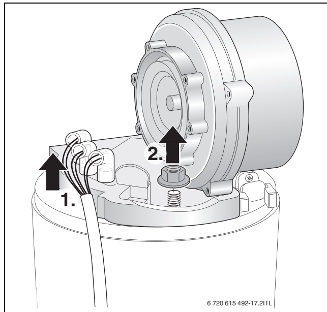
56. ábra A ventilátor kivétele
