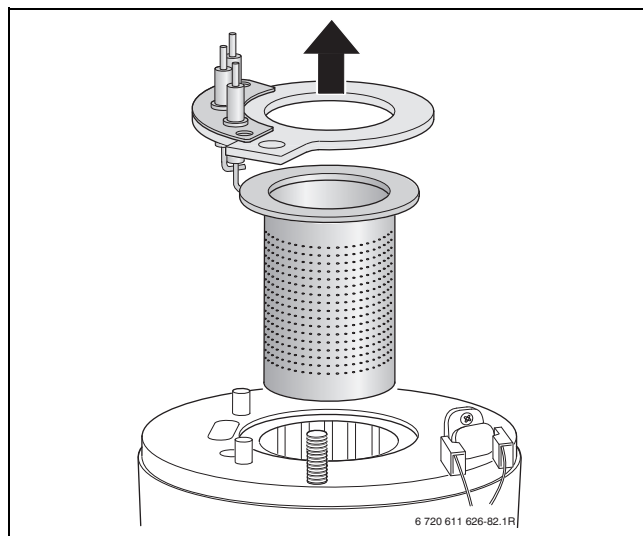
57. ábra Az égő kiserelése
