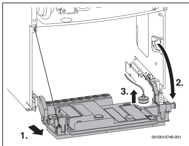
75. ábra A vezérlőelektronika lehajtása
