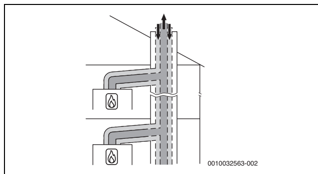
17. ábra Több fűtőkészülék bekötése a C (10) 3x szerint koncentrikus levegő-/füstgázvezetéssel a felállítási helyiségben
