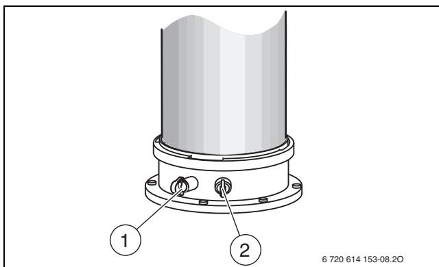
53. ábra Füstgáz-mérőcsonk és égésilevegő-mérőcsonk
