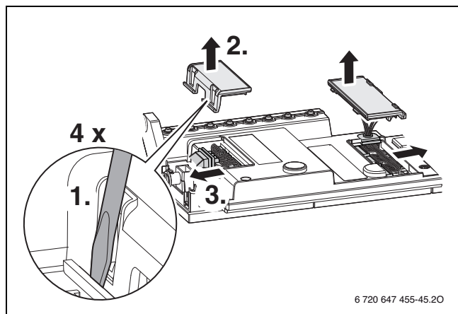
76. ábra Burkolat eltávolítása
