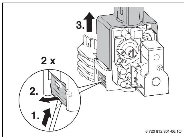
73. ábra Gázarmatúra kiserelése
