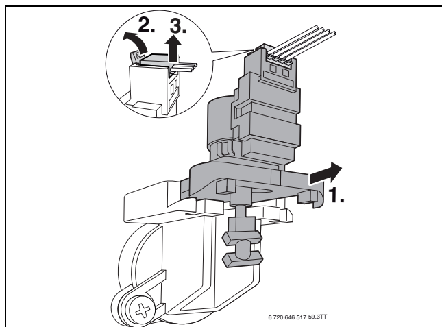
69. ábra Váltószelep motorjának kiserelése
