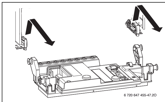
77. ábra Válassza le a vezérlőelektronikát.
