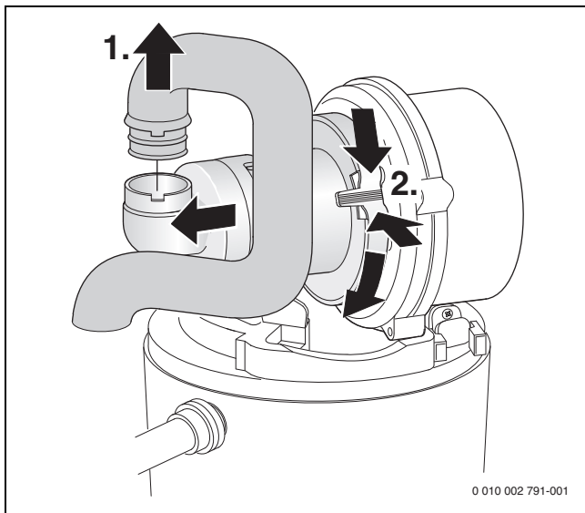
55. ábra A szívócső és az előkeverő kiserelése
