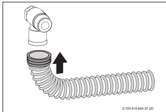
25. ábra A tömlő felszerelése a biztonsági szelepre
