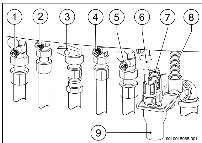
29. ábra Gáz- és vízőldali csatlakozások (külön rendelhető tartozékok)
