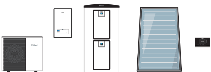
aroTHERM plus + VWZ MEH 97 hidraulikus állomás, allSTOR exclusiv multifunkciós puffer frissvizes- és szolár állomással, auroTHERM plus napkollektor, sensoCOMFORT
